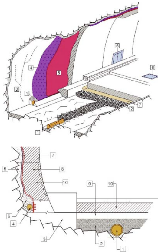
Figura 1: Sistema Paraguas incluyendo detalles del drenaje
