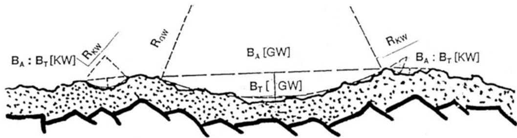
Figura 2: Criterios para el hormigón proyectado
